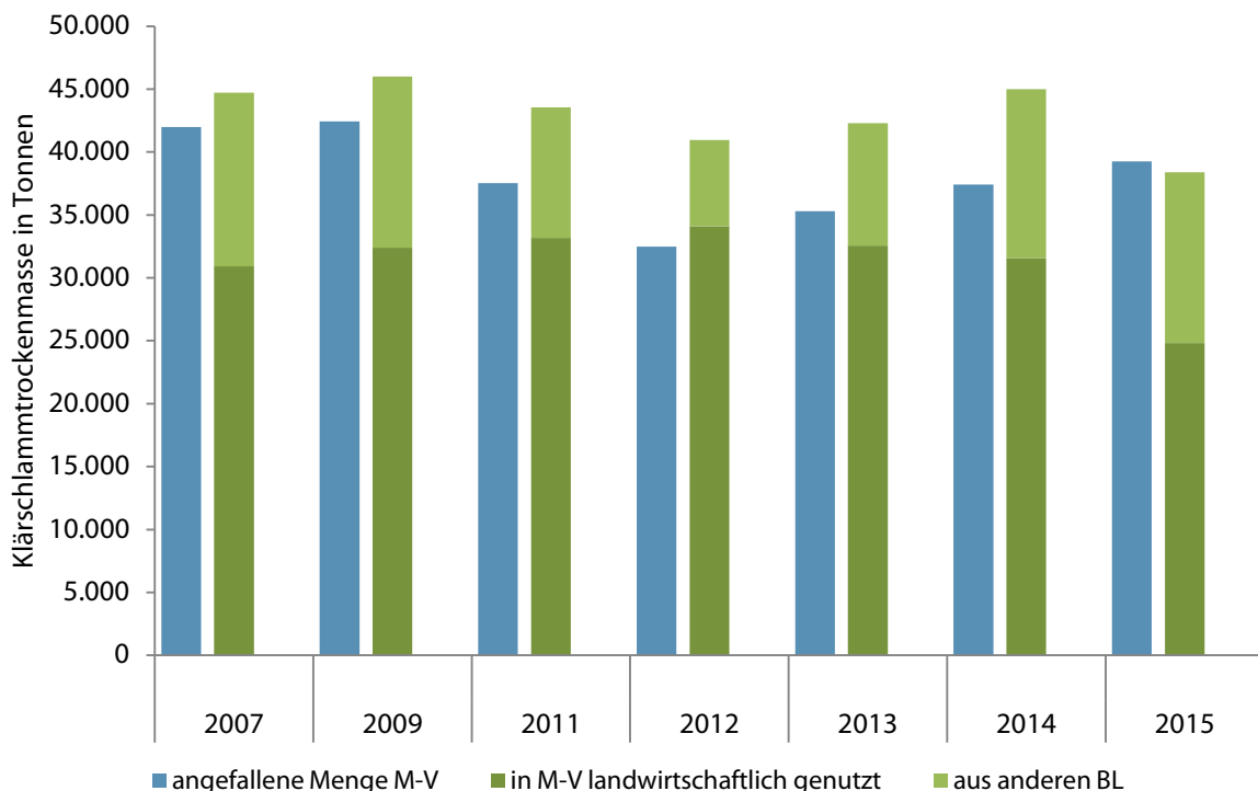
Abbildung 3-1: Klärschlammaufkommen und landwirtschaftliche Verwertung
