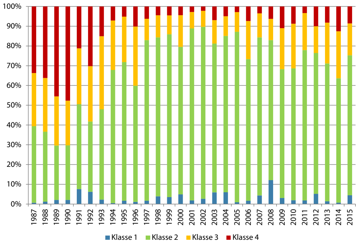
Abbildung 1-2: Klassifizierung der Wasserqualität anhand von Orthophosphat-Phosphor nach LAWA [27]
